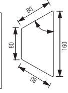
Arbeitsplatte B 80/160 x H 3 x T 69 cm
