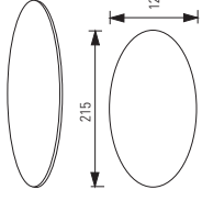
Arbeitsplatte B 215 x H 3 x T 120 cm
